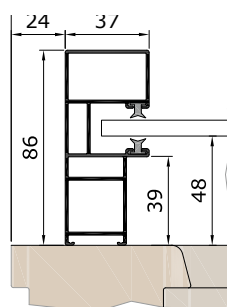
Führungsschiene KD37K
