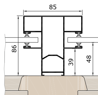
Führungsschiene KD85K
