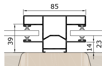
Führungsschiene KE85K
