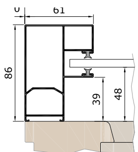
Führungsschiene KD61K
